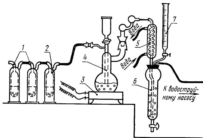
1—склянка-ловушка с серной кислотой; 2—склянка-ловушка с водой; 3—электролитка; 4—дистилляционная колба типа Кьельдаля из термостойкого стекла вместимостью 500 мл с пришлифованной пробкой, снабженной капельной воронкой с краном; 5—холодильник; 6—сосуд для улавливания аммиака; 7—микробюретка
